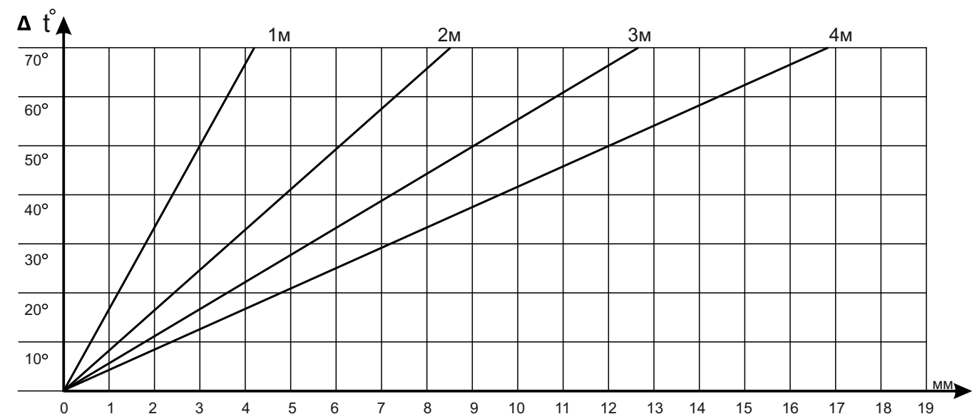
Линейное расширение трубопровода PBK (PP-R/GF/PP-R)
